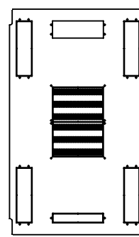
Omara 19" 80120 odprtine za uvod kablov stranske: 90 x 290 mm zadaj: 90 x 290 mm spredaj: 50 x 290 mm
