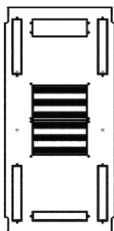
Omara 19" 60120 odprtine za uvod kablov stranske: 50 x 290 mm zadaj: 90 x 290 mm spredaj: 50 x 290 mm
