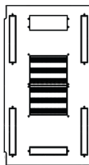
Omara 19" 70120 odprtine za uvod kablov stranske: 50 x 290 mm zadaj: 90 x 290 mm spredaj: 50 x 290 mm
