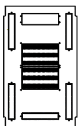
Omara 19" 60100 odprtine za uvod kablov stranske: 50 x 290 mm zadaj: 90 x 290 mm spredaj: 50 x 290 mm
