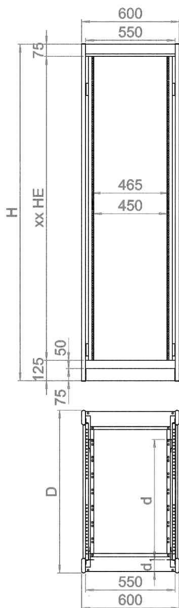
Slika tloris 60100
