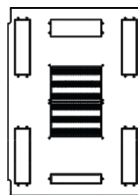
Omara 19" 80100 odprtine za uvod kablov stranske: 90 x 290 mm zadaj: 90 x 290 mm spredaj: 50 x 290 mm
