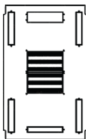
Omara 19" 70100 odprtine za uvod kablov stranske: 50 x 290 mm zadaj: 90 x 290 mm spredaj: 50 x 290 mm
