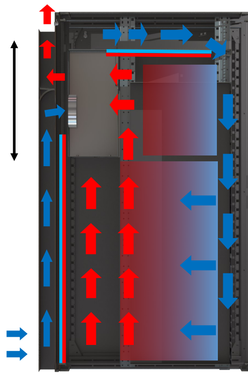
Schema vgrajene opreme
