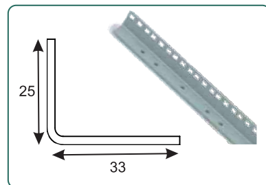
Profil 19" Net
