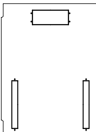
Omara 19" 80100 odprtine za uvod kablov zadaj: 90 x 290 mm ob strani: 50 x 290
