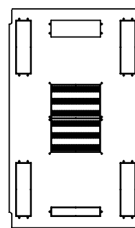
Omara 19" 80120 odprtine za uvod kablov stranske: 90 x 290 mm zadaj: 90 x 290 mm spredaj: 50 x 290 mm
