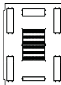
Omara 19" 80100 odprtine za uvod kablov stranske: 90 x 290 mm zadaj: 90 x 290 mm spredaj: 50 x 290 mm
