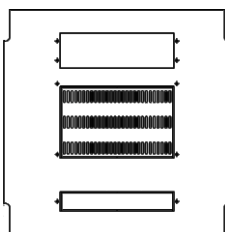
Omara 19" 6060 odprtine za uvod kablov zadaj: 90 x 290 mm spredaj: 50 x 290 mm
