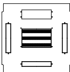
Omara 19" 7070 odprtine za uvod kablov stranske: 50 x 290 mm zadaj: 90 x 290 mm spredaj: 50 x 290 mm
