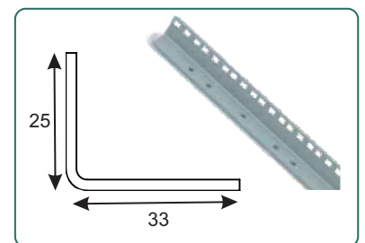
Profil 19" Net
