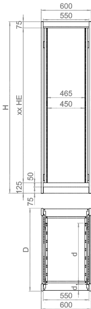
Slika toris 60100
