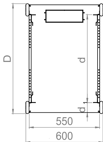
Slika tloris 60800
