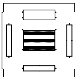
Omara 19" 7070 odprtine za uvod kablov stranske: 50 \times 290 mm zadaj: 90 \times 290 mm spredaj: 50 \times 290 mm
