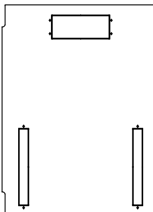
Omara 19" 80100 odprtine za uvod kablov zadaj: 90 x 290 mm ob strani: 50 x 290
