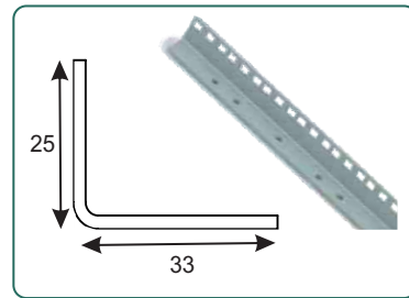
9" profil Net
