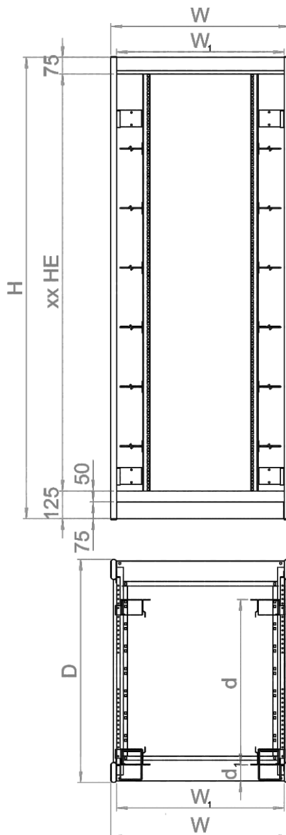
Slika toris 80100
