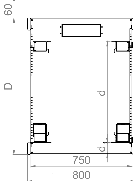
Slika tloris 80100
