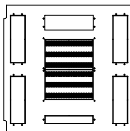
Omara 19" 8080 odprtine za uvod kablov stranske: 90 \times 290 mm zadaj: 90 \times 290 mm spredaj: 50 \times 290 mm
