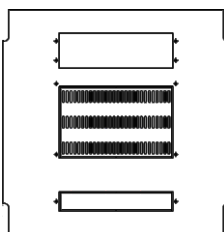
Omara 19" 6060 odprtine za uvod kablov stranske: 50 \times 290 mm zadaj: 90 \times 290 mm spredaj: 50 \times 290 mm
