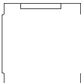
Omara 19" 60060 odprtine za uvod kablov zadaj: 50 x 290 mm
