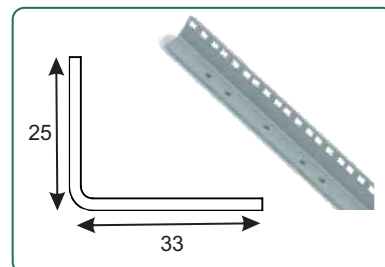
Profil 19" Net
