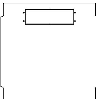
Omara 19" 60060 odprtine za uvod kablov zadaj: 90 x 290 mm
