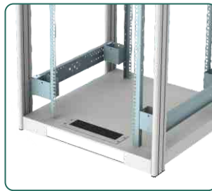
Uvod kablov zadaj pokrit s ščetko
