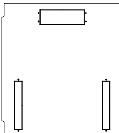
Omara 19" 80080 odprtine za uvod kablov zadaj: 90 x 290 mm spredaj ob strani: 50x290mm
