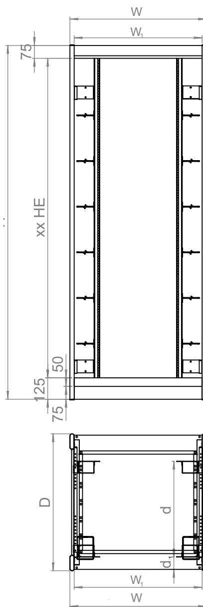
Slika tloris 8080
