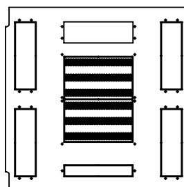
Omara 19" 8080 odprtine za uvod kablov stranske: 90 x 290 mm zadaj: 90 x 290 mm spredaj: 50 x 290 mm
