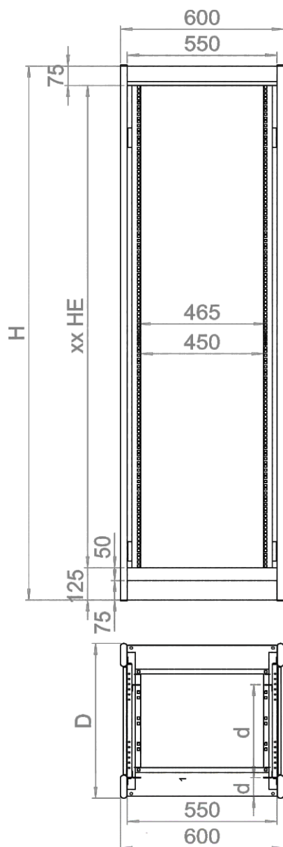
Slika tloris 6060
