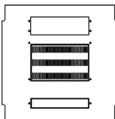
Omara 19" 6060 odprtine za uvod kablov stranske: 50 x 290 mm zadaj: 90 x 290 mm spredaj: 50 x 290 mm
